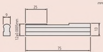
Скругленная губка : 619013
