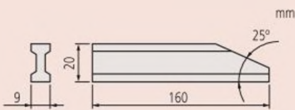
Плоская губка : 619018
